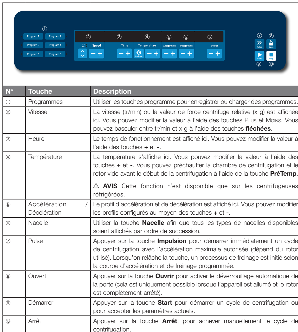
Figure 4–1: Fonctions du panneau de commande LCD
